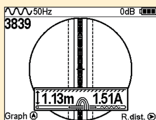
Автоматическое измерение глубины и силы тока
